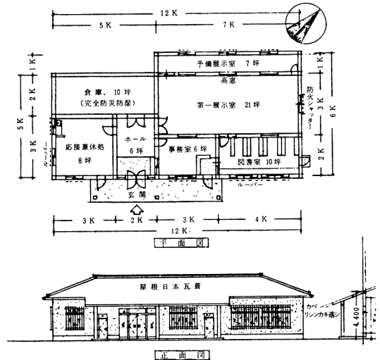
新しき村美術館第一次建設案 (74坪)
